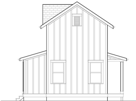
RIGHT ELEVATION
